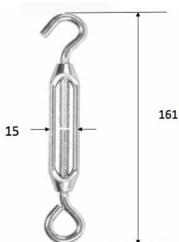
TENSOR DE GANCHO CON ARMELLA \frac{7}{32}" \times 6\frac{3}{8}"
