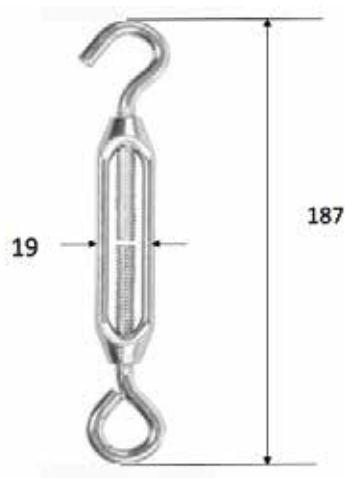
TENSOR DE GANCHO CON ARMELLA \frac{1}{4}" \times 7\frac{3}{8}"
